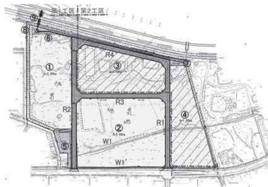
▲工業団地土地利用計画図
